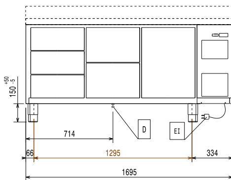
Front aanzicht
